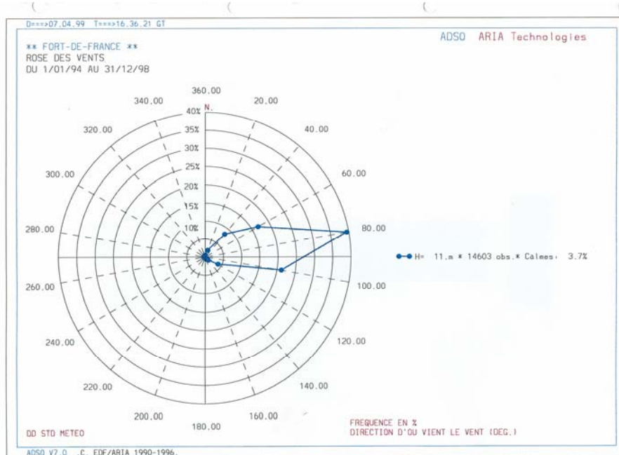
Figure 1. Rose des vents générale de la station de Fort-de-France (aéroport Le Lamentin)
