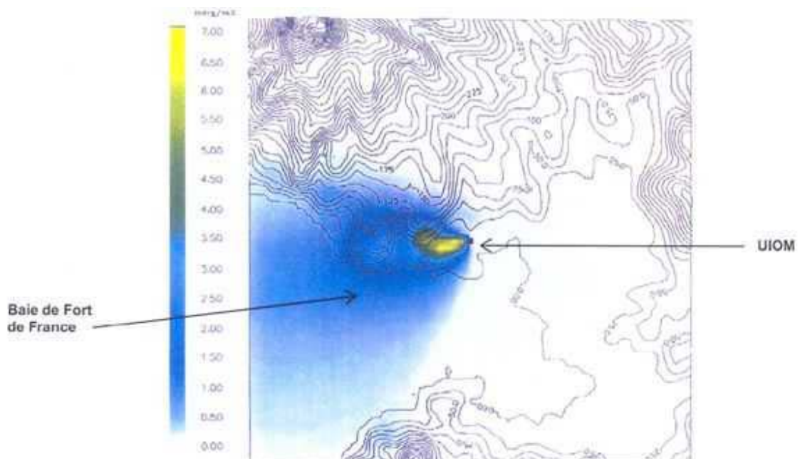
Figure 2. Concentration en moyenne annuelle pour les NOx
